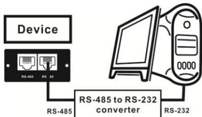
Korzystanie z konwertera RS-485 na RS-232
