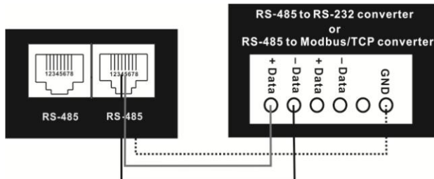
Połączenie przewodowe między RJ45 a konwerterem mediów
