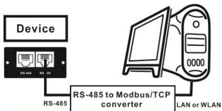
Użyj konwertera RS-485 na Modbus/TCP
