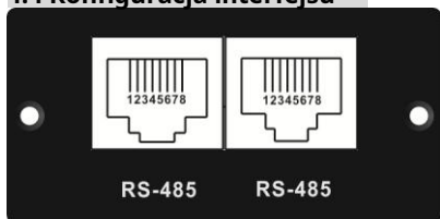
Konfiguracja pinów RS-485
