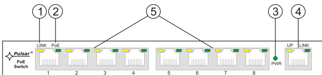
Rys.4. Widok Switch'a.
