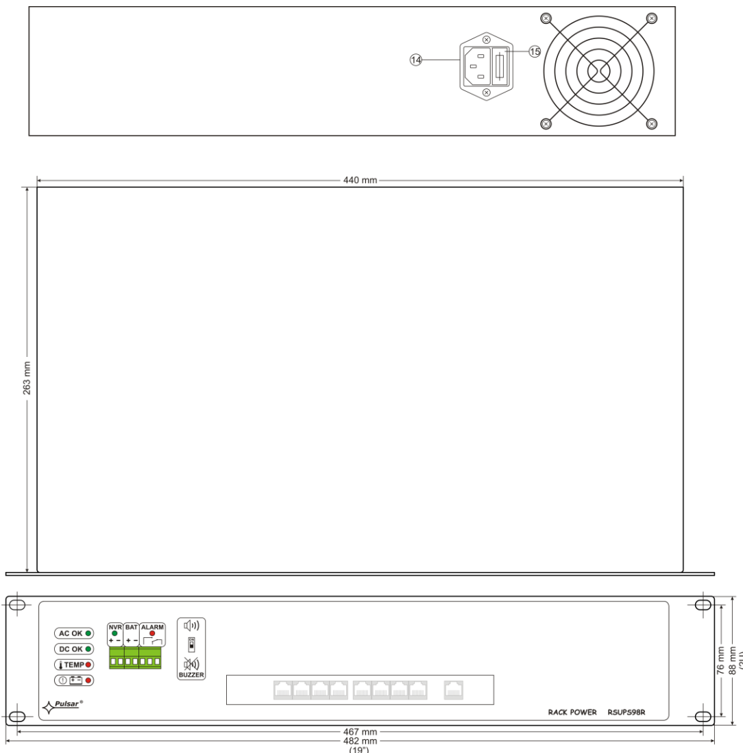
Rys.3. Widok zasilacza.
