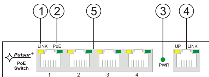
Rys.4. Widok Switch'a.
