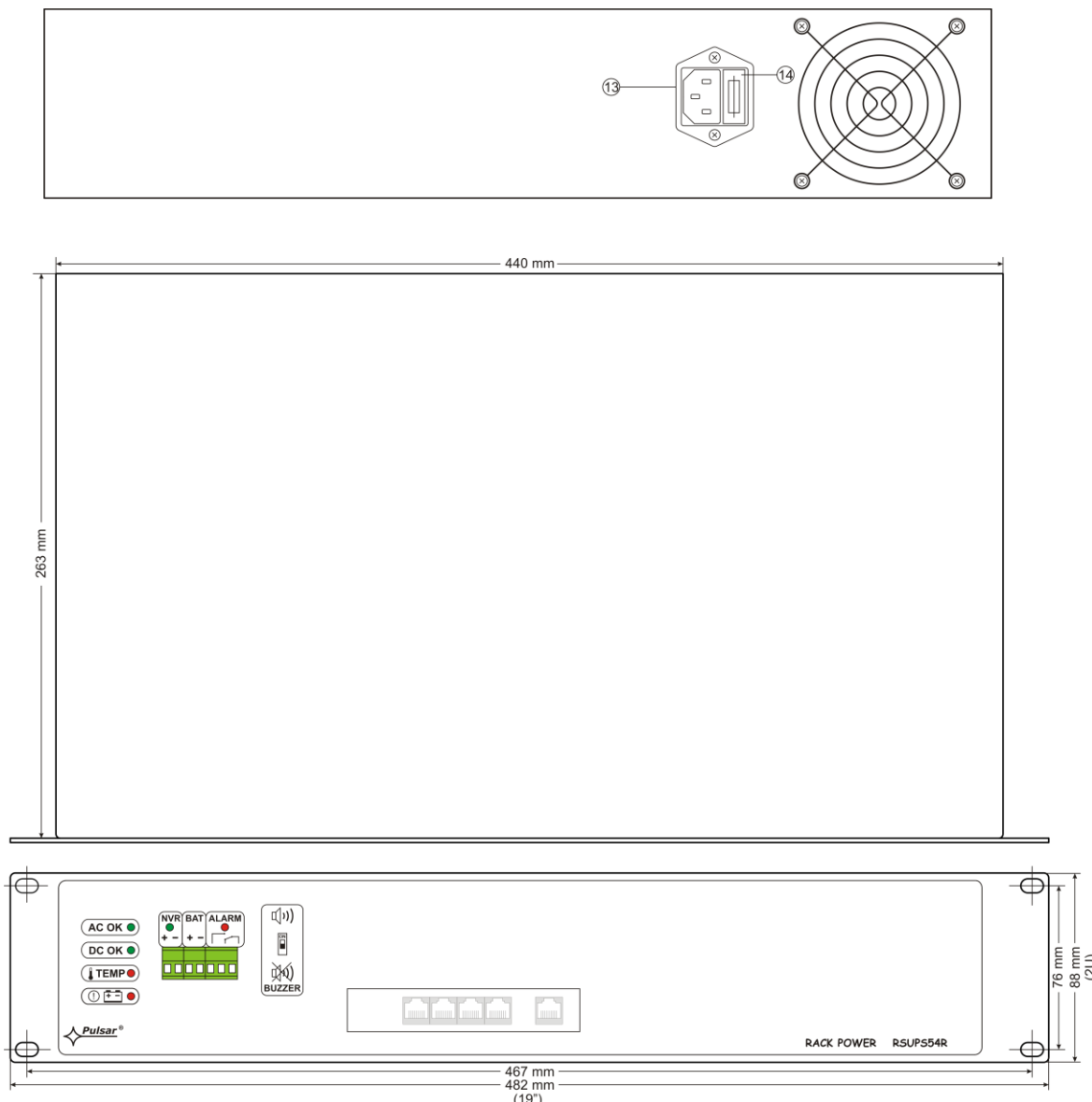
Rys.3. Widok zasilacza.
