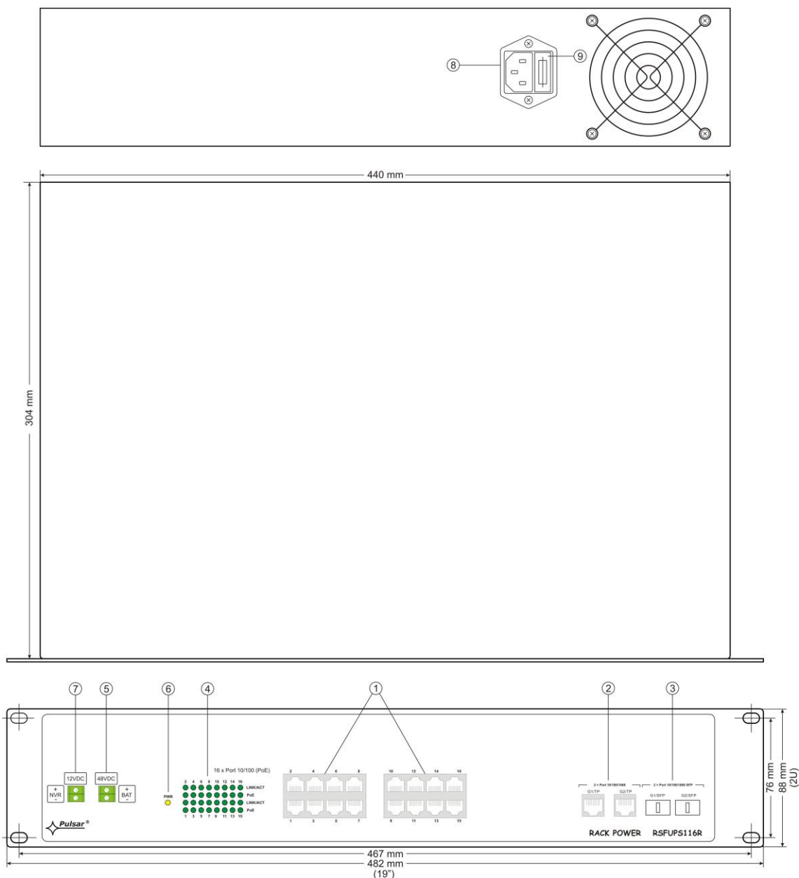
Rys.2. Widok obudowy.
