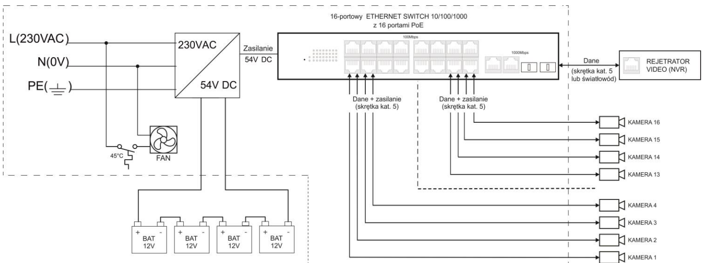
Rys. 1. Schemat blokowy.
